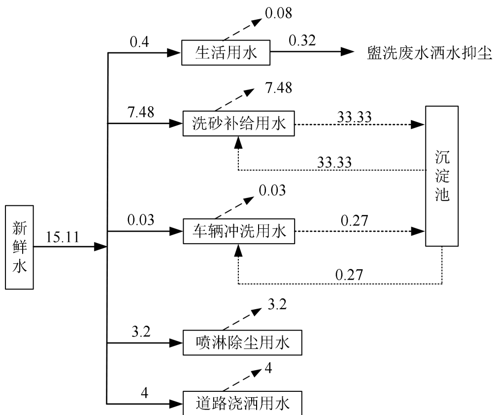
图2 本项目水平衡图 (单位: \text{m}^3/\text{d} )
