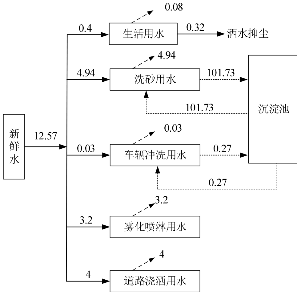
图2 本项目水平衡图 (单位: m 3 /d)
